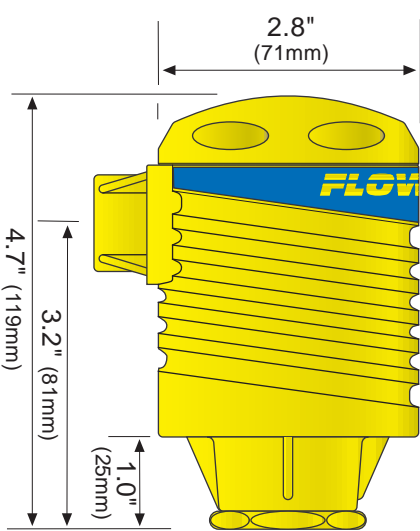
LC05 Dimensions
