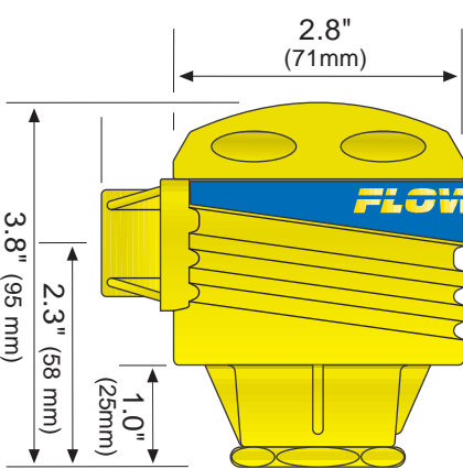
LC06 Dimensions
